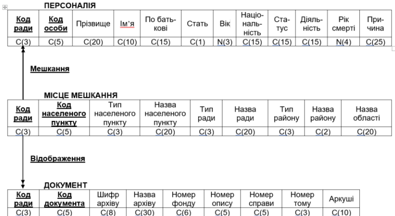
Рис. 4. Даталогічна модель БД
