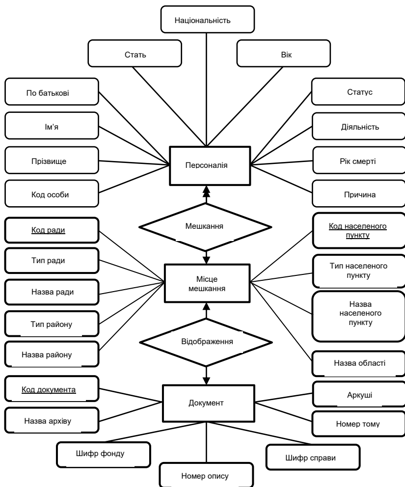
Рис. 3. Глобальна ER-діаграма БД
