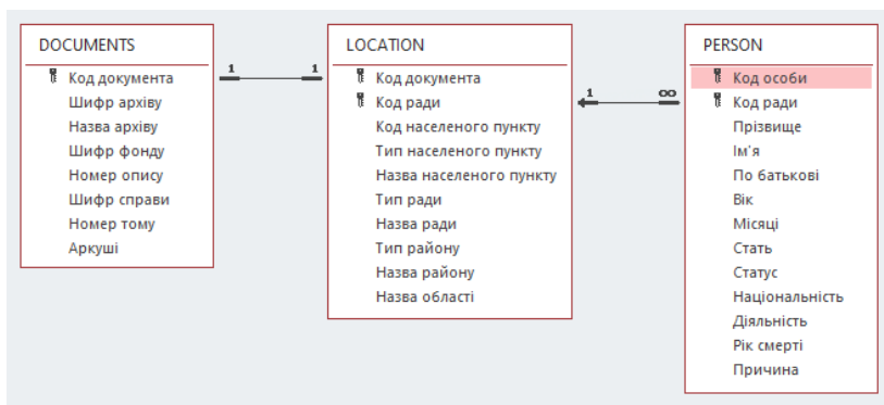
Рис. 5. Ілюстрація схеми даних фізичної реалізації БД
