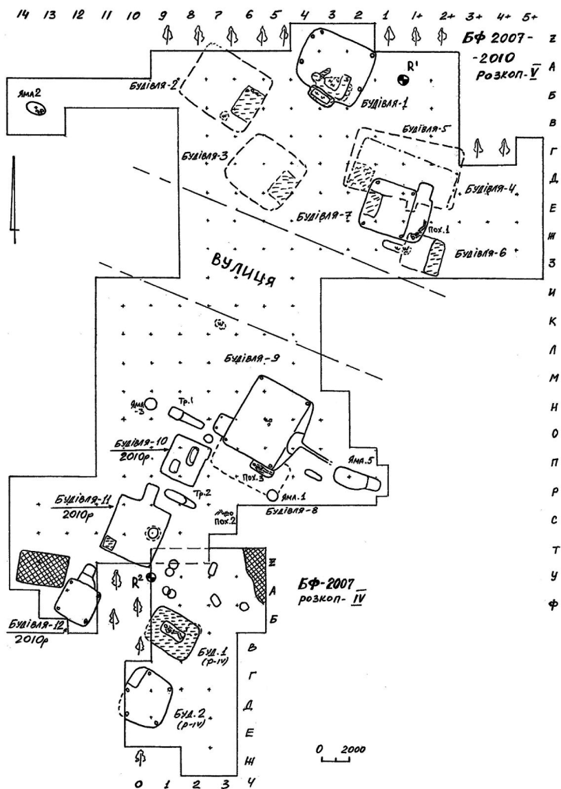
Рис. 1. План розкопу V із позначенням відкритих у 2010 р. нерухомих об'єктів
