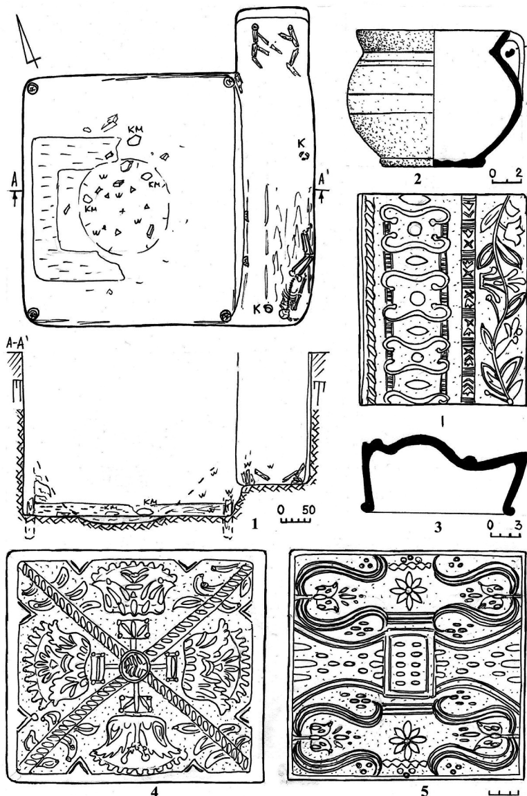
Рис. 2. Землянка № 7 розкопу V та знахідки з неї: 1 – план землянки; 2 – келих; 3 – 5 – пічні кахлі
