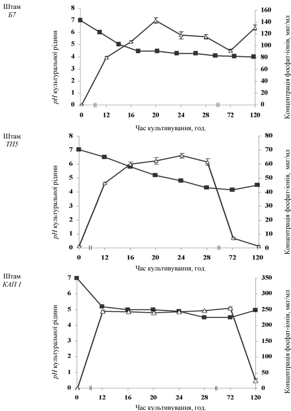
Рис. 3. Динаміка концентрації фосфат-іонів і pH культуральної рідини у виділених штамів фосфатмобілізуючих бактерій
