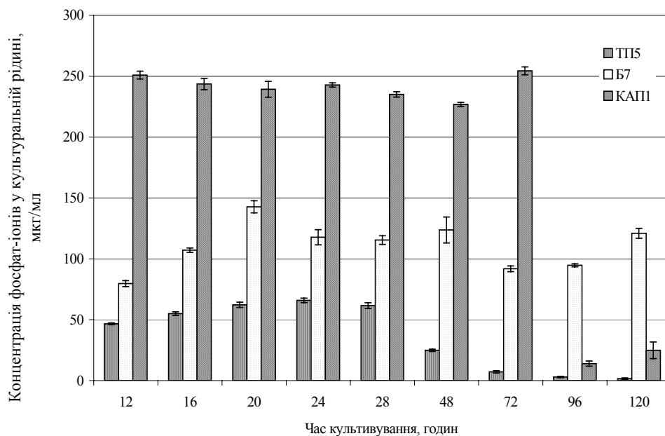
Рис. 1. Динаміка накопичення фосфат-іонів у культуральній рідині виділених штамів фосфатмобілізуючих бактерій
