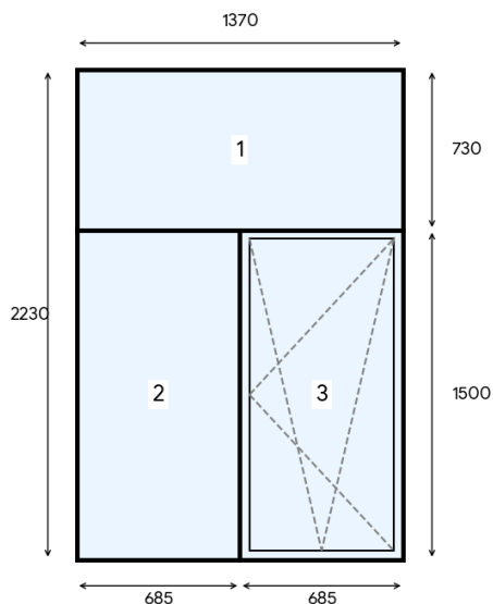
Вікно металопластикове (орієнтовний розмір 1370*2230мм)
