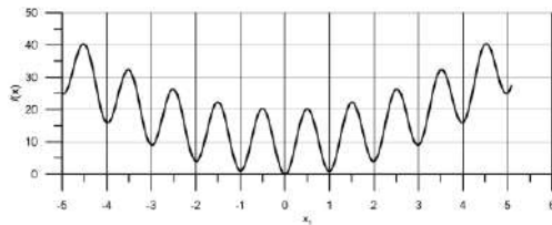
Рис. 1. Багатоекстремальність. Функція Растрігіна
