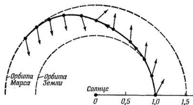
Рис. 1б) Траєкторія польоту
