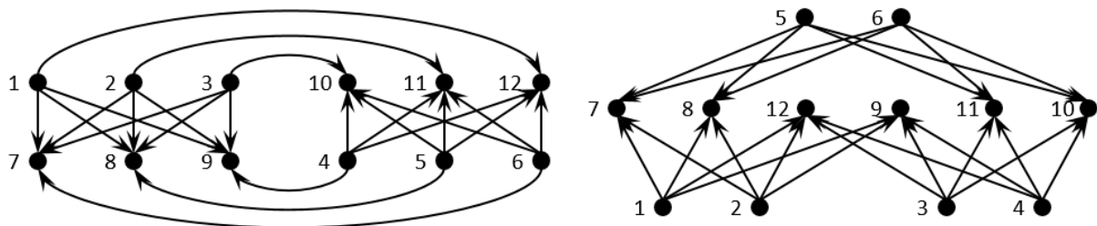
Рис. 1. Двогранні графи з різними довжинами оптимальних упорядкувань при h = 4
